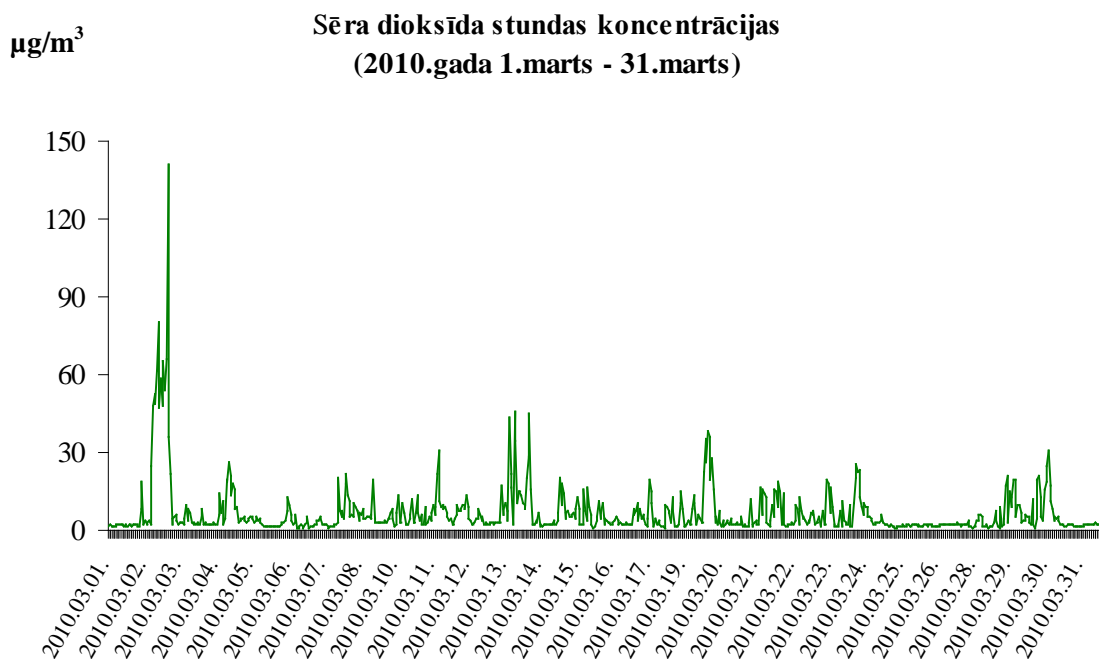
4.attēls. SO_2 stundas koncentrācijas stacijā BLB.
