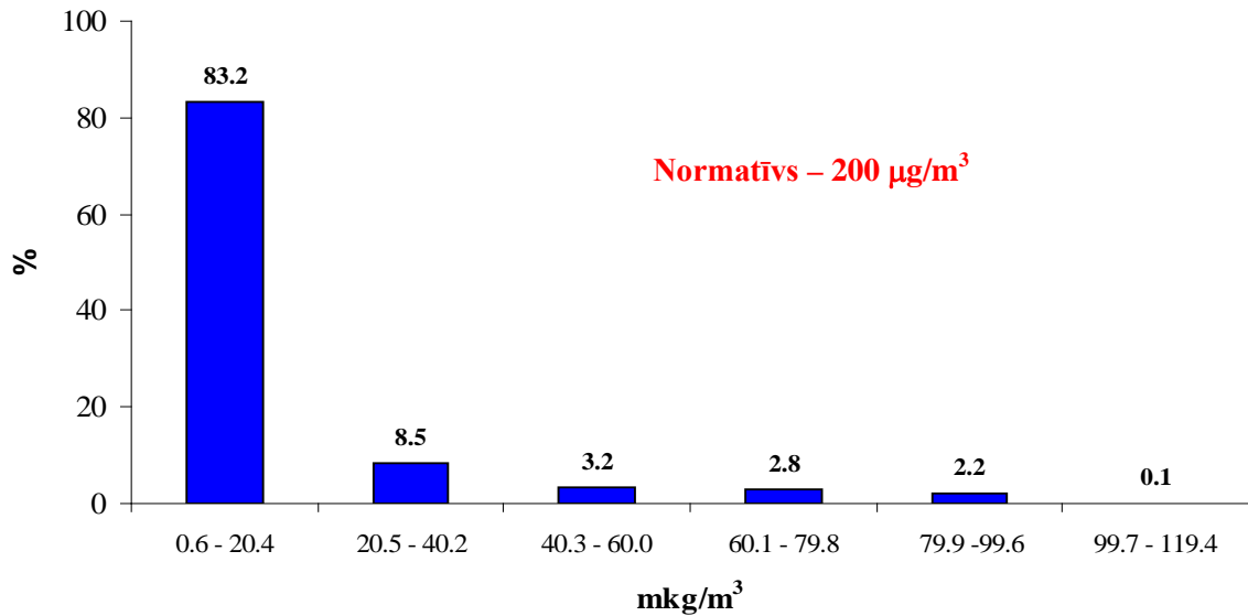
3. attēls. NO_2 stundas koncentrāciju ( \mu\text{g}/\text{m}^3 ) sadalījums stacijā Man-Tess.
