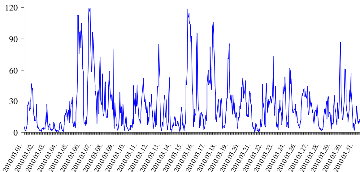
Slāpekļa dioksīda stundas koncentrācijas (2010. gada 1.marts - 31. marts)
